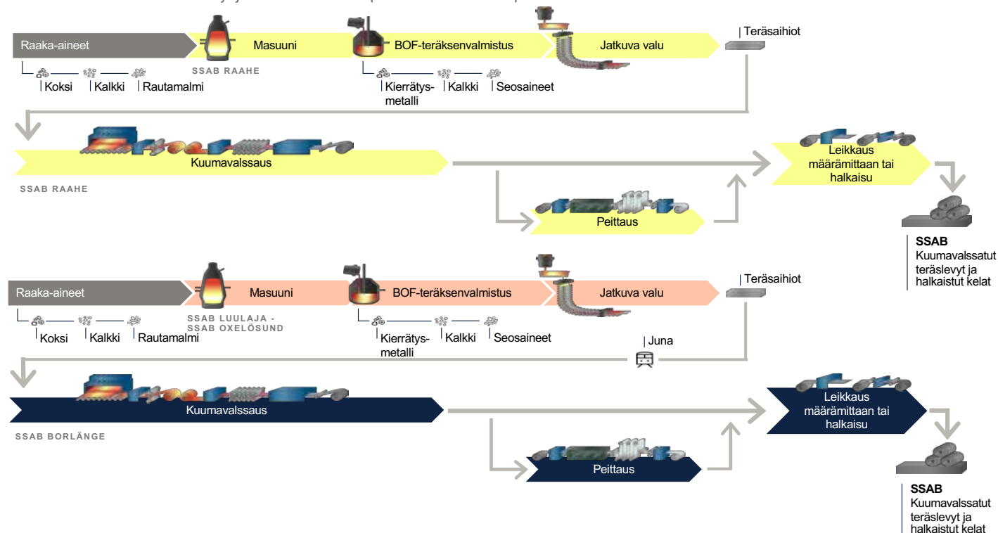
KUVA 1. SSAB:n tuotantolaitokset ja pääasialliset prosessivaiheet masuunipohjaisten kuumavalssattujen teräslevyjen ja halkaistujen kelojen valmistuksessa.
