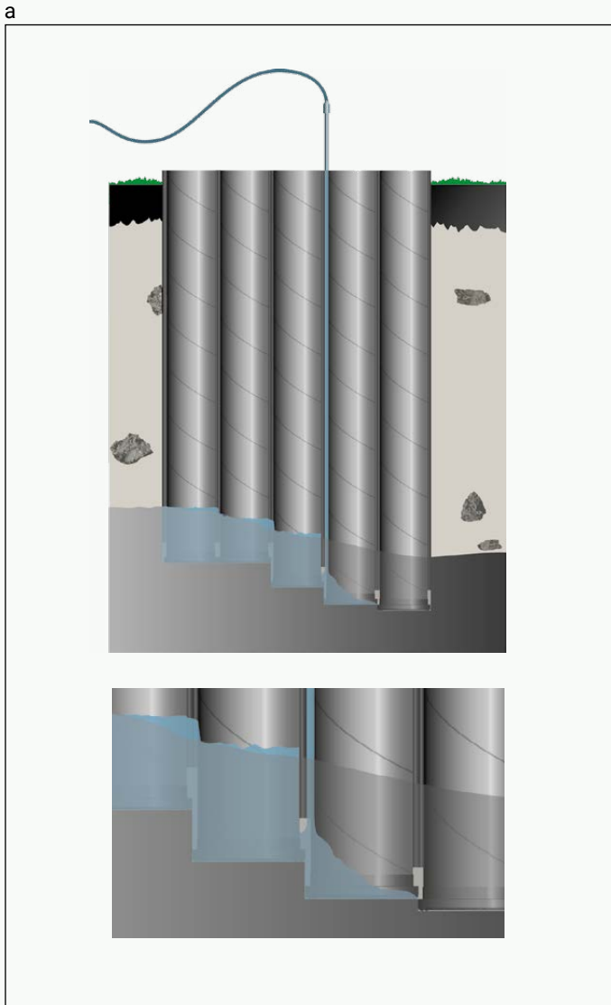
Kuva 20. RD-paaluseinän alapään ja taustan injektointi.
