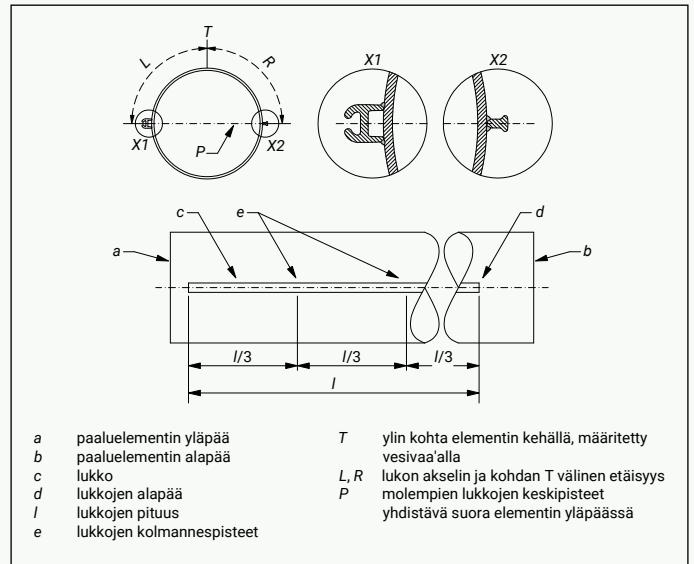
Kuva 28. Lukkojen toleranssien tarkistuspuisteiden sijainnit.
