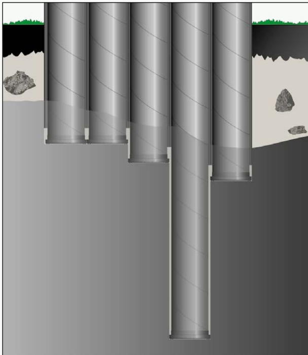
Kuva 30. Porattaessa RD-paalu edellistä paalua syvemmälle, ei leveä lukkoprofiili saa ulottua paalun kärkeen asti
