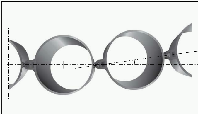
Kuva 17. Lukkoprofiilien asennuksella toteutettu lievä kulmamutoksesta johtuva poikkeama RD-paaluseinässä
