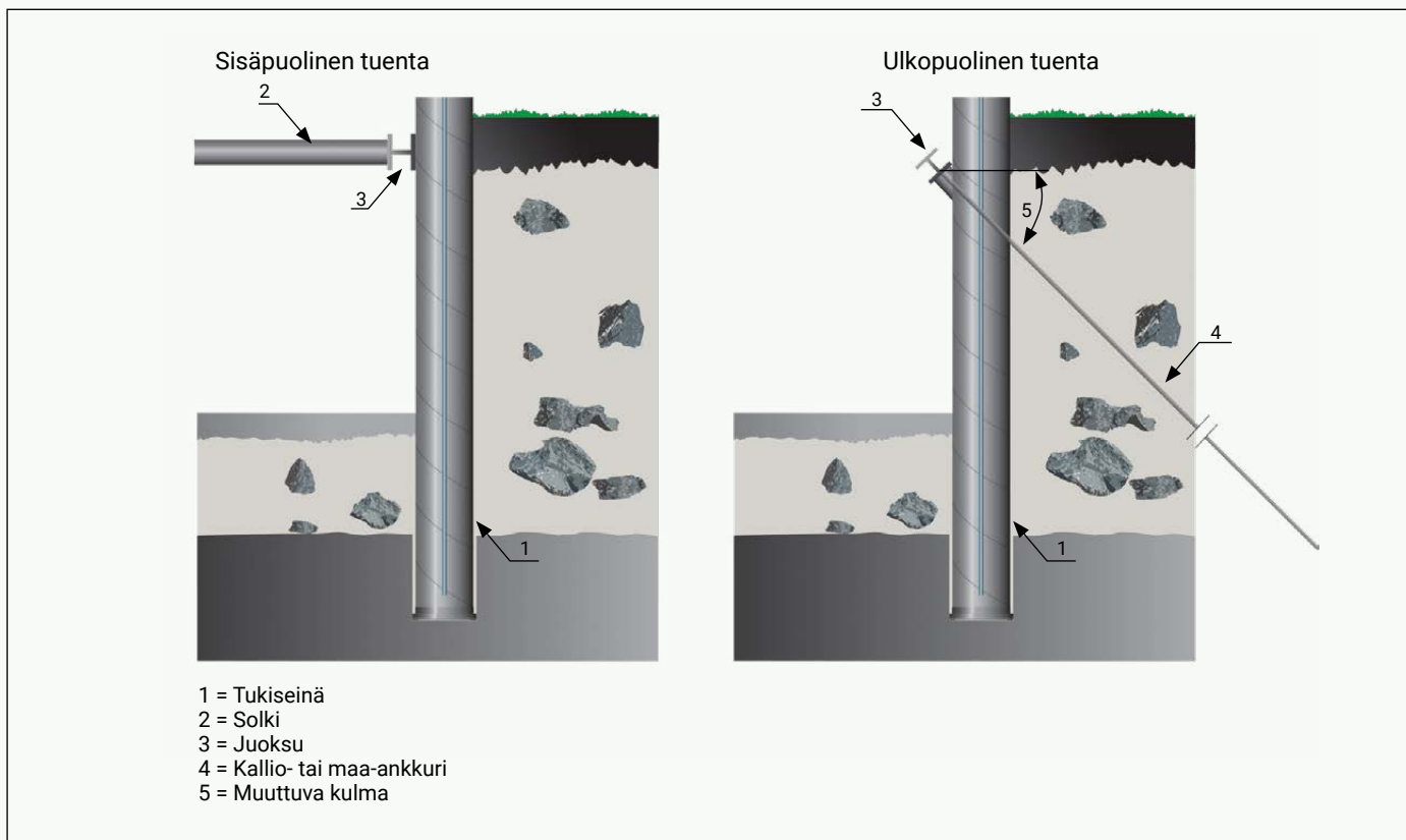
Kuva 21. RD-paaluseinän tuentatapoja
