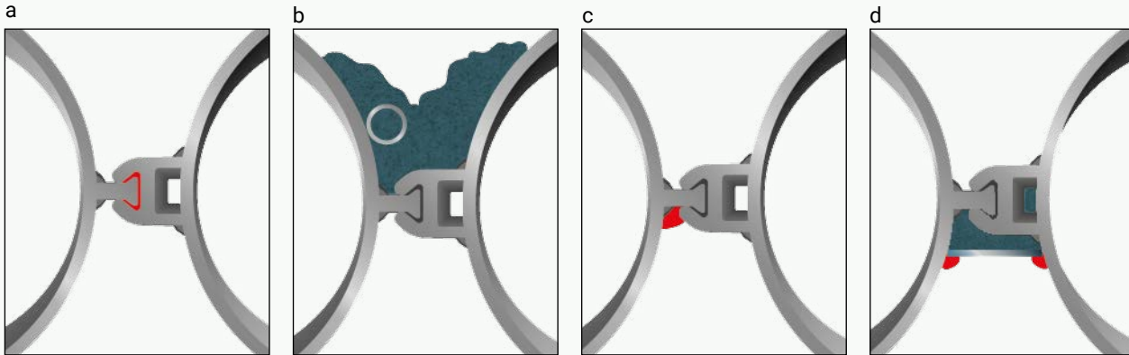
Kuva 18. RD-paaluseinän vesitiiviyden parantaminen lukkoprofiiliin asennettavalla tiivistysaineella (kuva a), taustan injektioinnilla (kuva b) ja vesitiiviyden varmistaminen hitsaamalla (kuvat c ja d).
