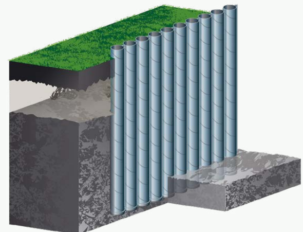
Kuva 5. RD-paaluseinä kallion sisään ulottuvana kaivannon tukiseinä
