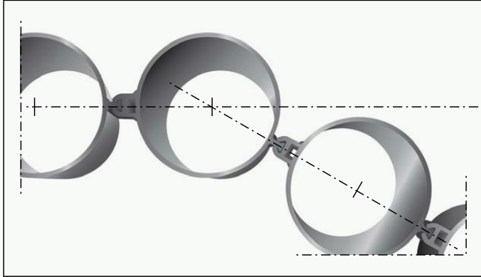
Kuva 16. Lukkoprofiilien asennuksella toteutettu suuri kulmamutoksesta johtuva poikkeama RD-paaluseinässä
