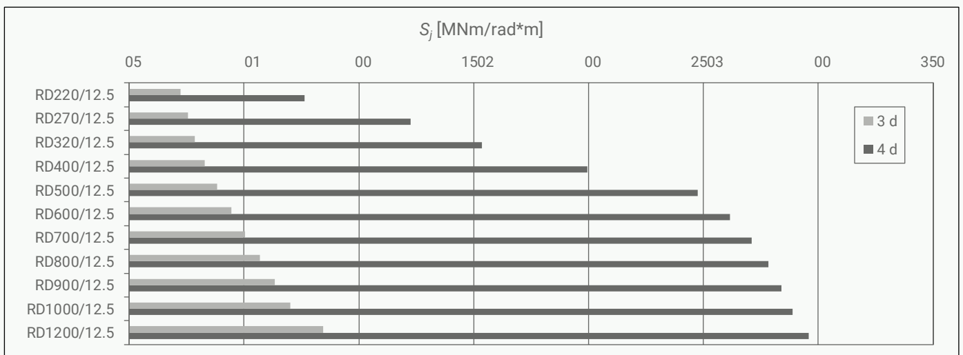
Kuva 14. RD-paaluseinän jäykkyys. Paalut RD220/12,5 ... RD1200/12,5, RM/RF-lukkoprofiilit. Poraussyvyudet 3-d ja 4-d ehjään kallioon. Injektointimassan nimellisluku C20/25.
