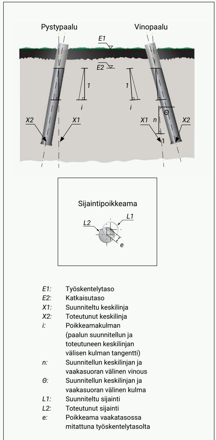
Kuva 31. Geometrinen rakentamistoleranssien määrittely
